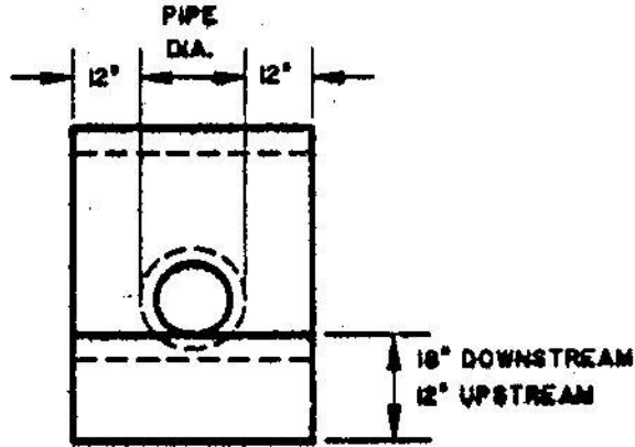
END ELEVATION
